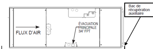
Installation horizontale du côté droit La rotation du bloc ventilateur n'est pas nécessaire.
