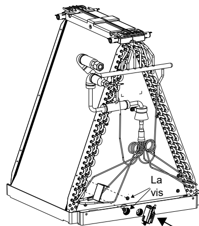
Capteur de fuite de frigorigène
